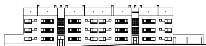
ALZADO NORTE
