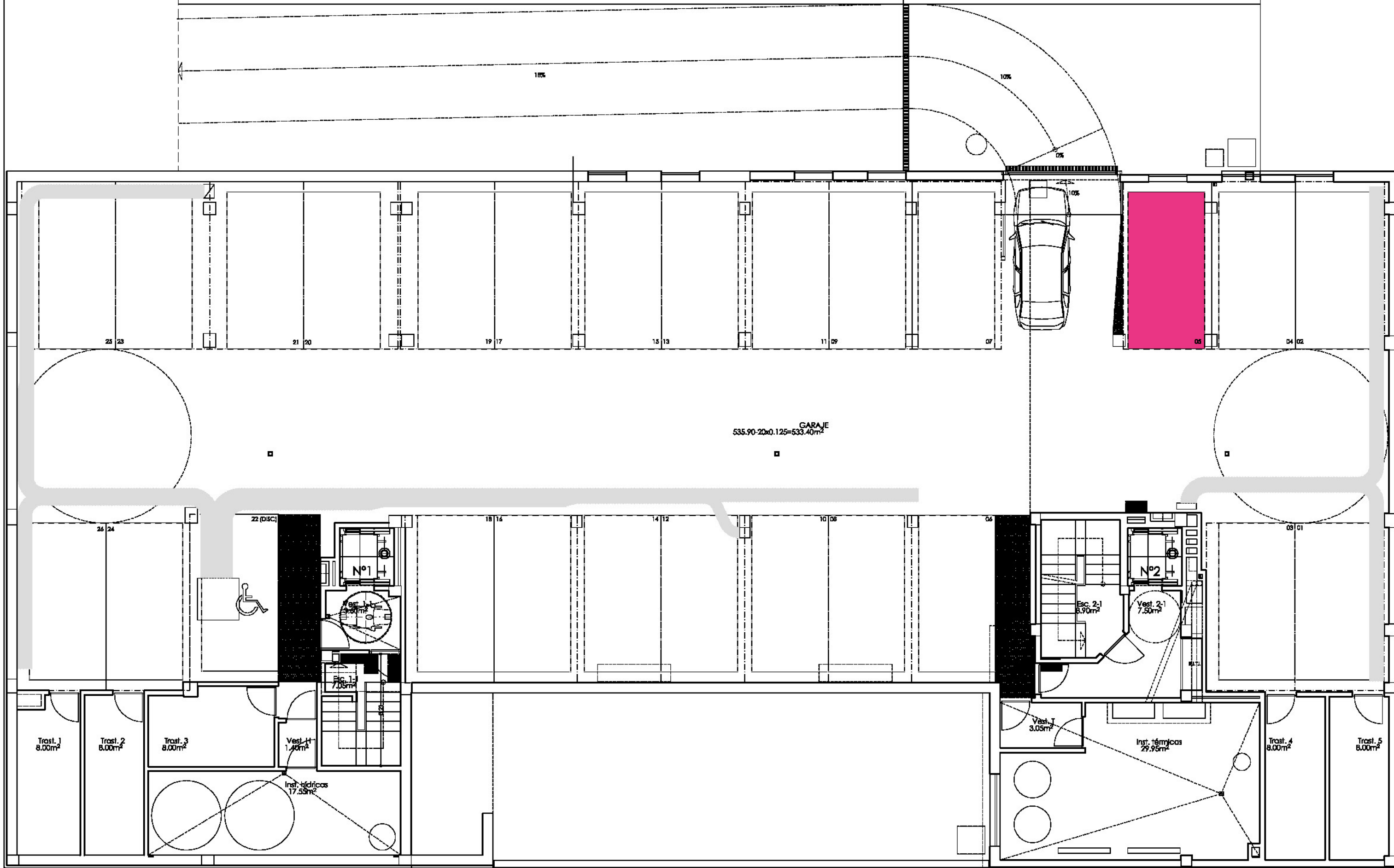
PLANTA SÓTANO -1
