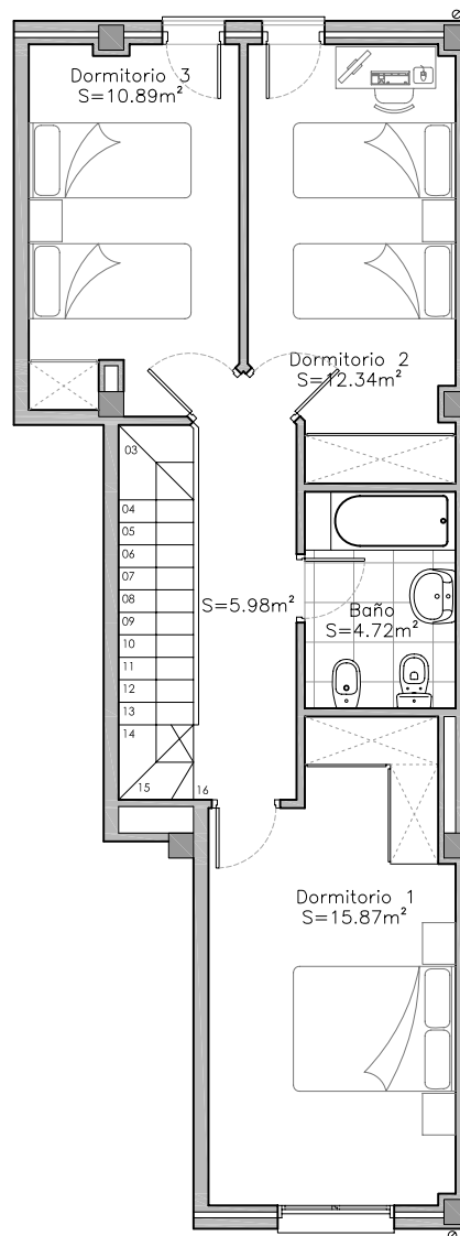
PLANTA PRIMERA
